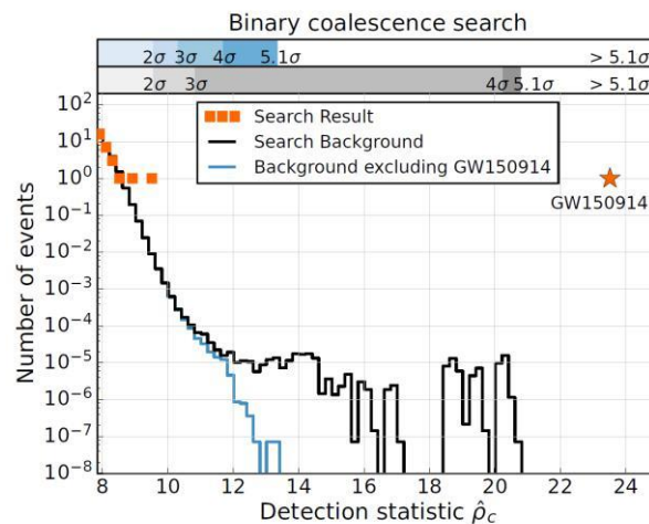
Figura 4. (Adaptada da Figura 4 da nossa publicação). Resultados da nossa pesquisa para a coalescência binário quantificando quão incomum é GW150914 em comparação com outros "eventos" falsos decorrentes de flutuações de ruído. Esta pesquisa concluiu que um evento de ruído imitando GW150914 seria extremamente raro - menos do que uma ocorrência em cerca de 200.000 anos - um valor que corresponde a um nível de significância de detecção de mais de cinco "Sigma".
