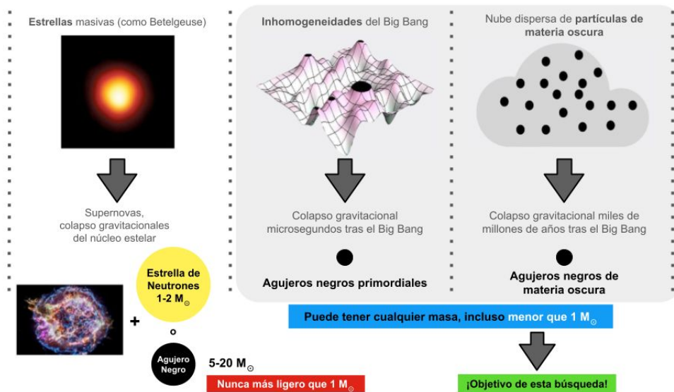
Figura 1: Esquema de los diferentes procesos que dan lugar a los objetos compactos que pueden observarse con LIGO-Virgo-KAGRA. Además de las estrellas de neutrones y los agujeros negros formados por evolución estelar, existen hipotéticos agujeros negros primordiales o de materia oscura que podrían existir en el universo y tener una masa inferior a la de nuestro Sol.
