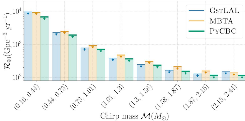
Figura 2: (Figura 5 en el artículo ): Límites superiores de la tasa de fusión de binarias de agujeros negros de masa subsolar, en función de la masa chirp, es decir, la suma de las masas de los dos agujeros negros que representa la masa efectiva del sistema binario. Estos límites superiores se deducen de la ausencia de detecciones en los datos de O4a y de la sensibilidad estimada de la búsqueda realizada por cada canal de análisis.
