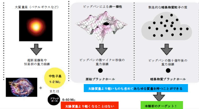
図 1: LVK 共同研究グループが検出するコンパクト天体の、考えられる形成経路を示した図。標準的な恒星進化は中性子星やブラックホールを生み出すが、太陽より軽いブラックホールを生み出すとは考えられていない。一方、初期宇宙で生成された原始ブラックホールや、いわゆる散逸性暗黒物質モデルで形成されるブラックホールなど、他の仮説的なメカニズムによって太陽質量以下のブラックホールが形成される可能性がある。
