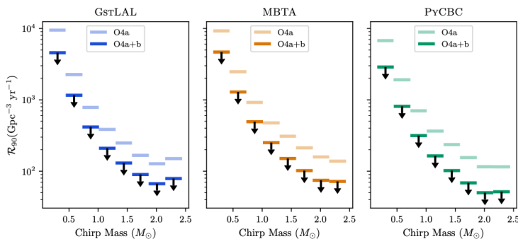
図2: (論文の図7) チャープ質量の関数として示した、少なくとも1つの太陽質量以下の天体を持つ連星ブラックホール母集団の合体率に対する信頼水準90%の上限値 ( R_{90} , 単位は1立方ギガパーセクあたり年間の件数)。O4aとO4bの結果を組み合わせることで、「O4a+b」と表記される合体率の統合推定値が得られている。3つの図それぞれにおいて、濃い(薄い)線はO4a+b(O4aのみ)解析の結果を示す。矢印は、O4a+b探索によって制約されない合体率の方向を示す。
